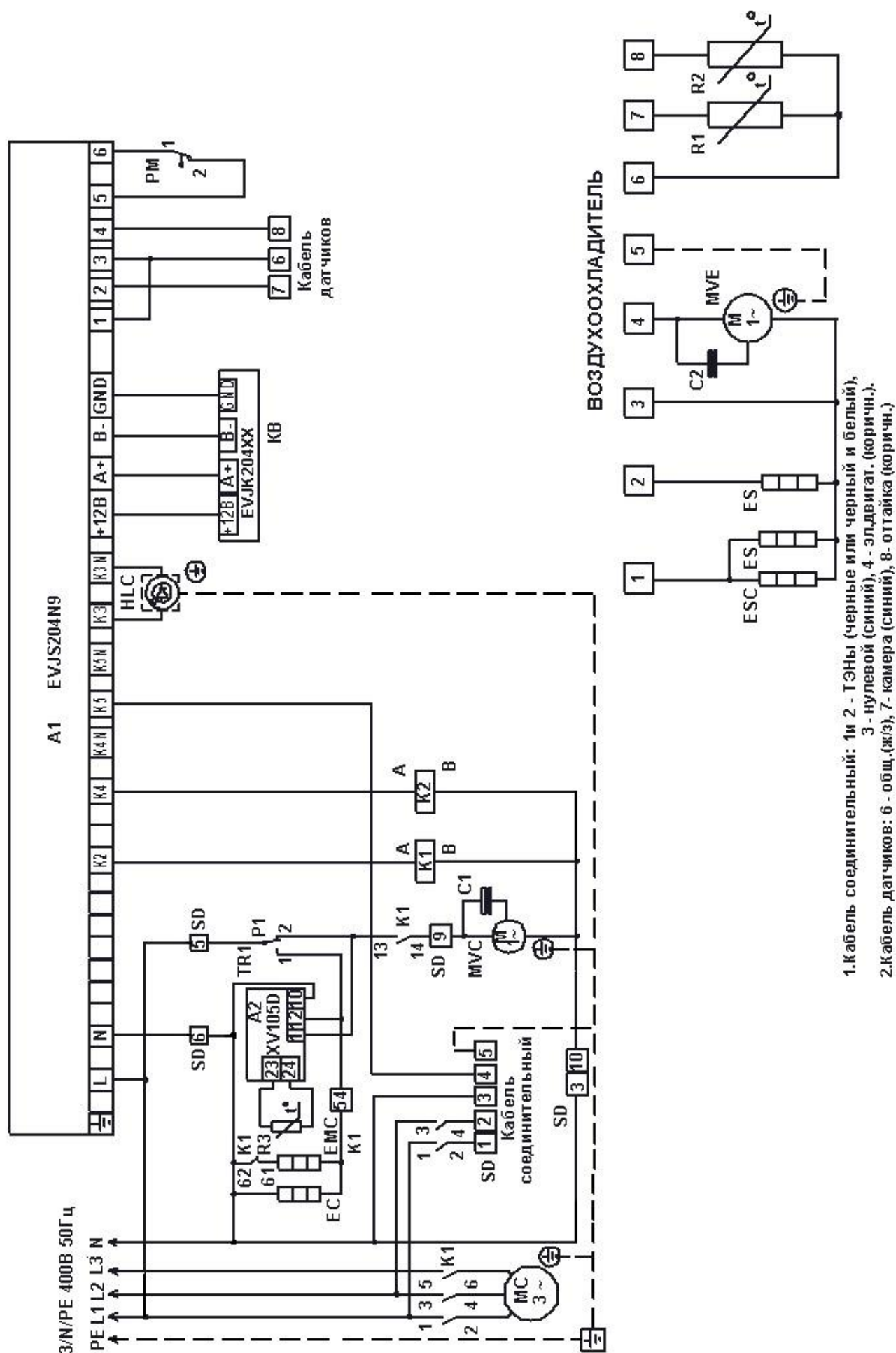
Рис.12 Схема электрическая принципиальная сплит-систем SM3...SDU,SB3...SDU.
