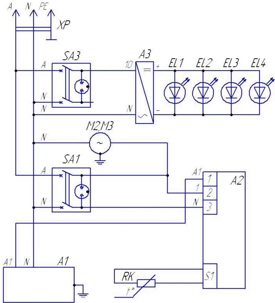
Схема электрическая принципиальная.
