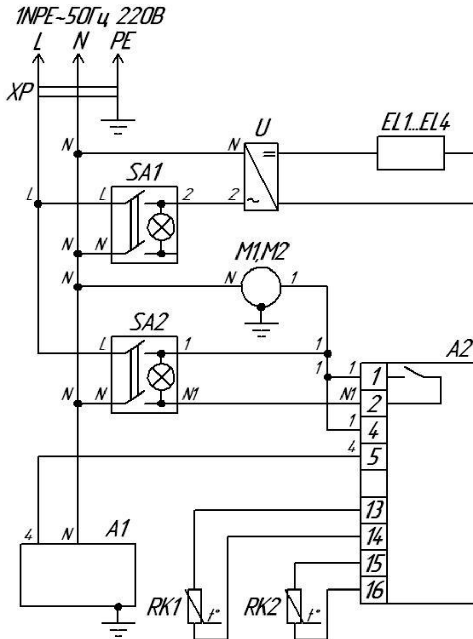
A1 - компрессорно-конденсаторный блок; A2 - контроллер; EL1...EL4 – светодиодная лента; M1,M2 - вентилятор; RK1,RK2 – датчик температуры; SA1 - выключатель освещения; SA2 - выключатель контроллера; U - источник питания для светодиодной ленты; XP - шнур питания с вилкой.
