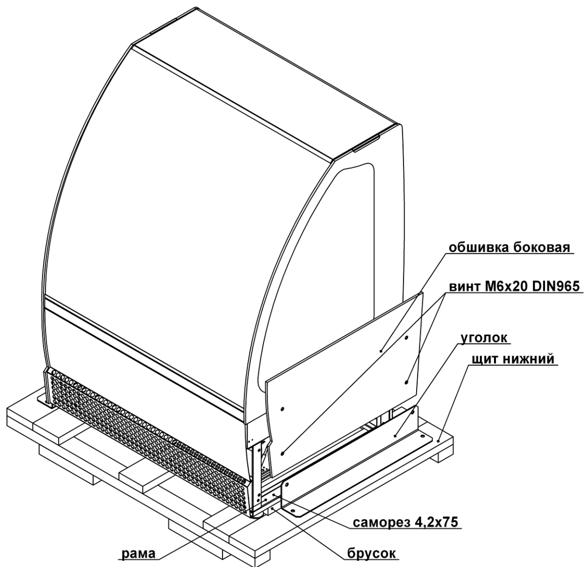
Схема распаковки VS/VSo
