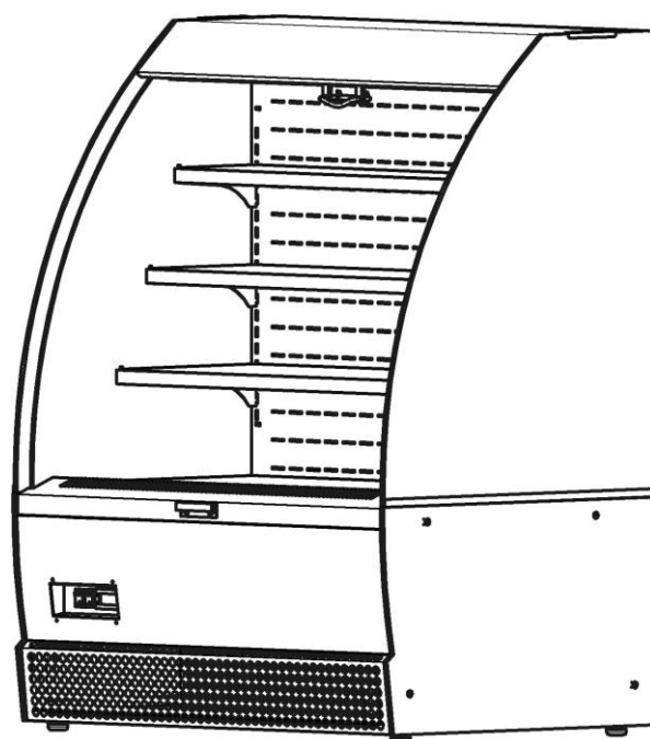
Схема сборки VSo-0,95GK / 1,3GK
