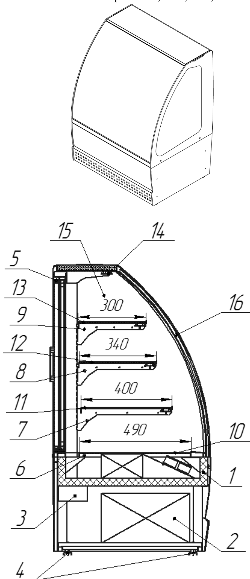
Схема сборки VS-0,75/-0,95/-1,3
