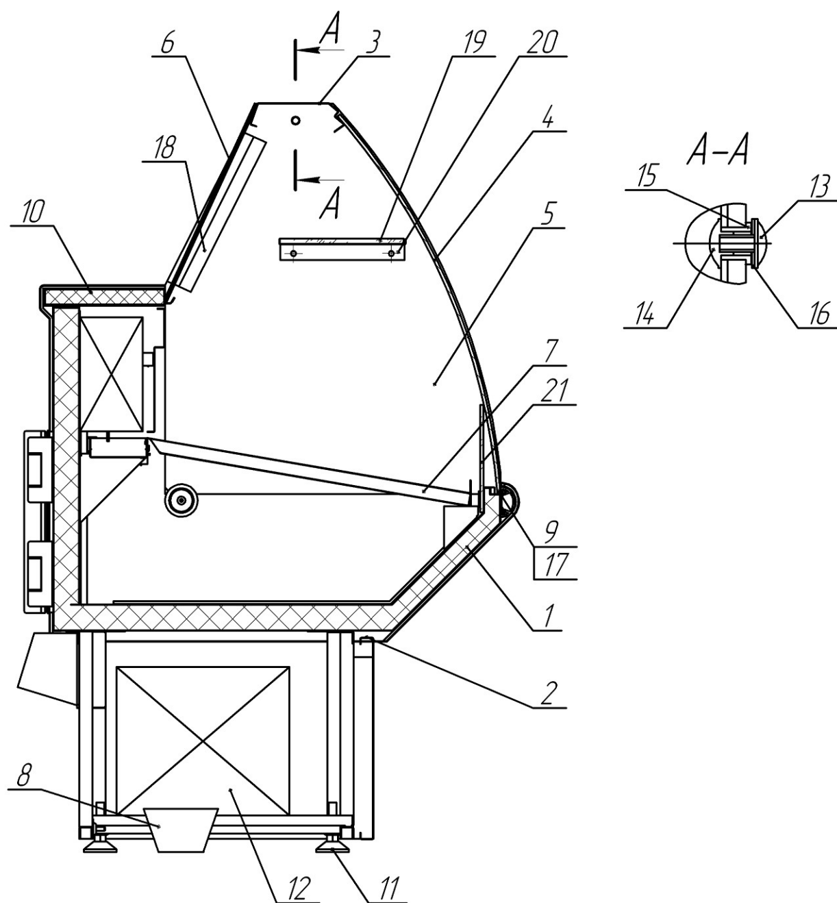
Схема сборки ВХС и ВХСн с радиусным стеклом
