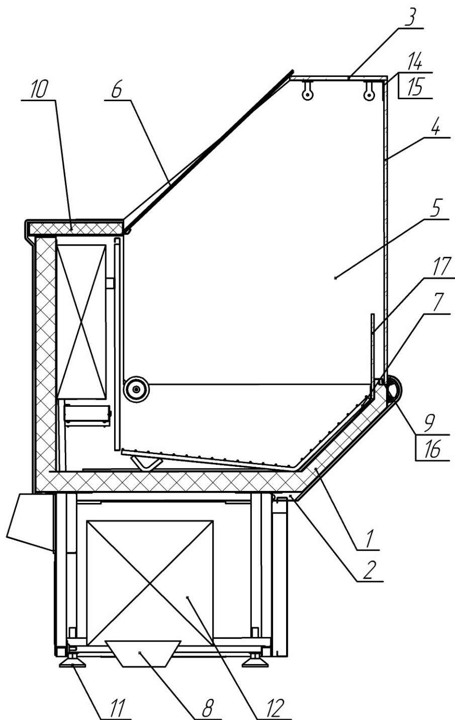
Схема сборки ВХН с прямым стеклом
