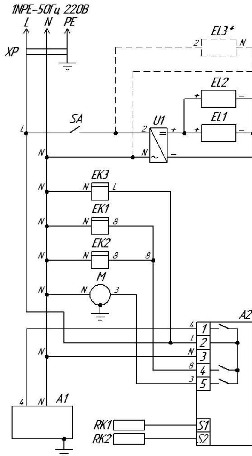
Схема электрическая принципиальная.
