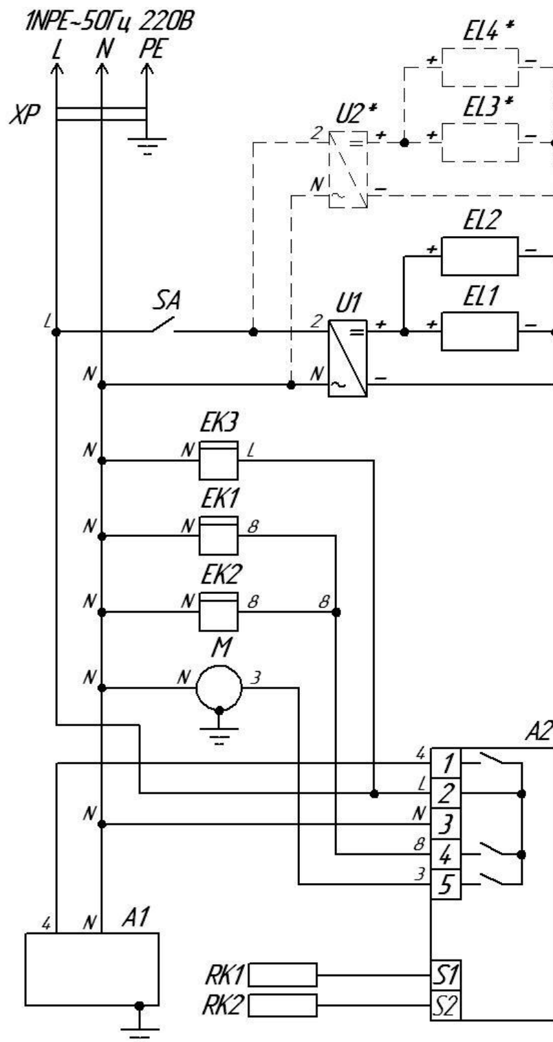
Схема электрическая принципиальная.
