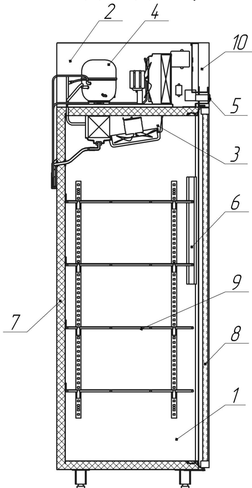
Разрез шкафа 0,5СКВ; 1,12СКВ; 1,12СКВ купе
