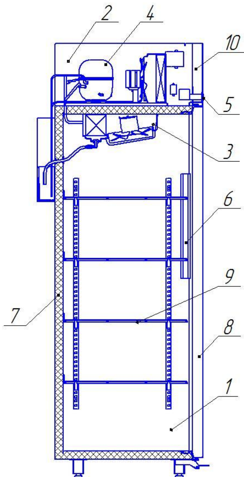
Разрез шкафа 0,5МВ; 0,7МВ; 0,7УМВ; 1,12МВ; 1,5МВ; 0,5Н; 0,7Н; 1,12Н; 1,5Н
