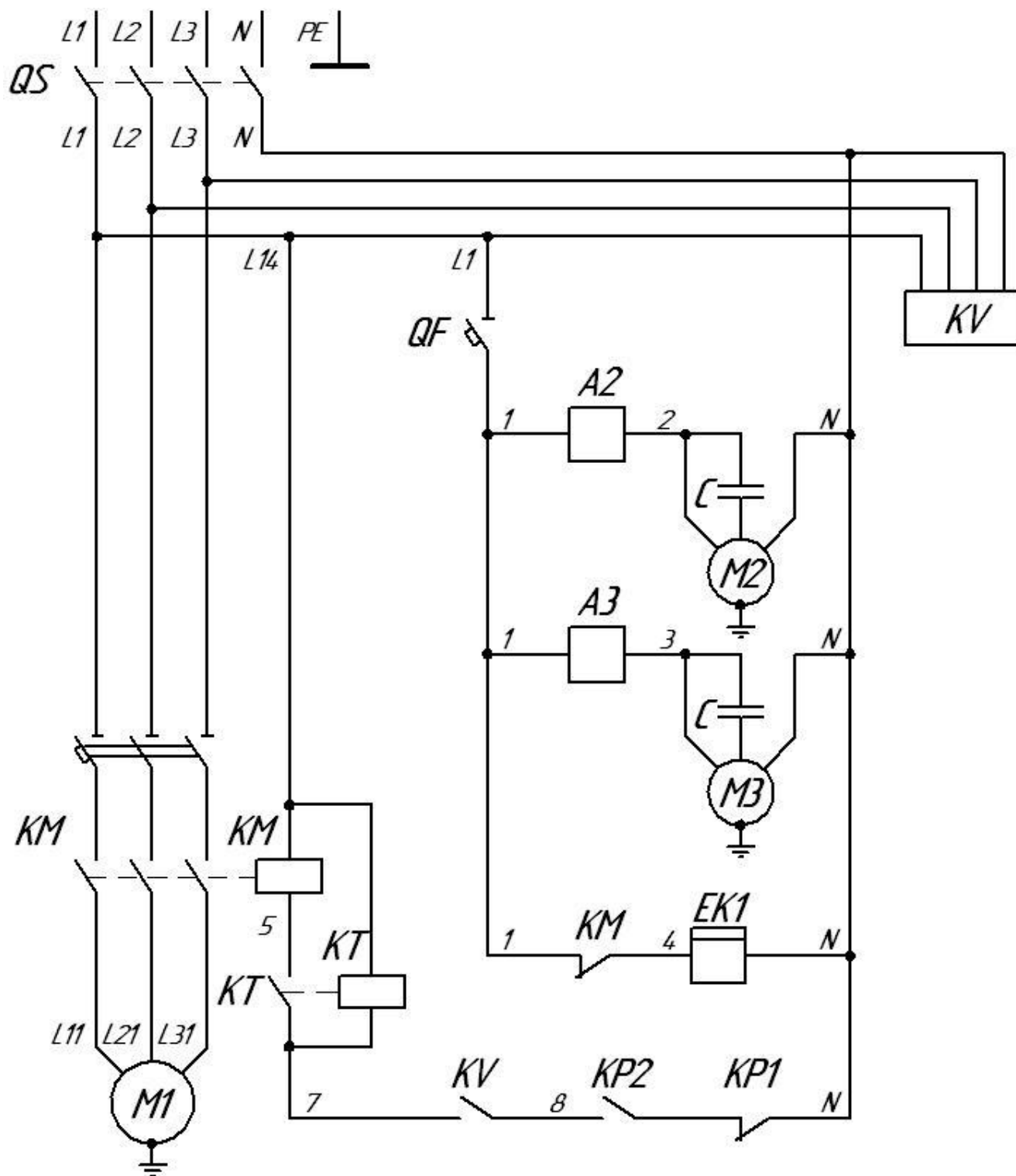
Схема электрическая принципиальная агрегатов с двумя вентиляторами
